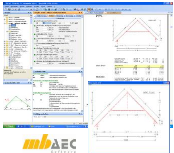
Auszug aus dem Eingabeprogramm und Darstellung eines statischen Systems eines Kehlbalkendachstuhl.
